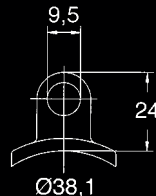
Tube Plate Art. nr S743A
