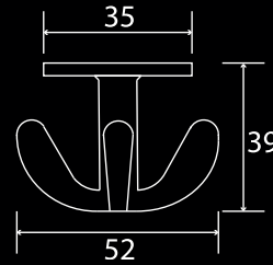
Robe Hook 860C
