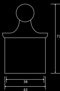
End Cap 736ACHS
