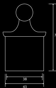
End Cap 736ACH
