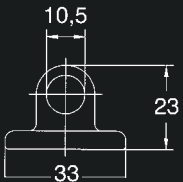
Hook Plate Art. nr S742A
