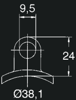
Tube Plate Art. nr S743A
