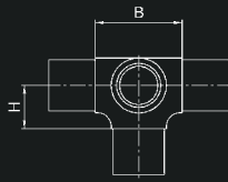
Flush Side Outlet Tee 90°
