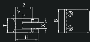
Glas Clip
